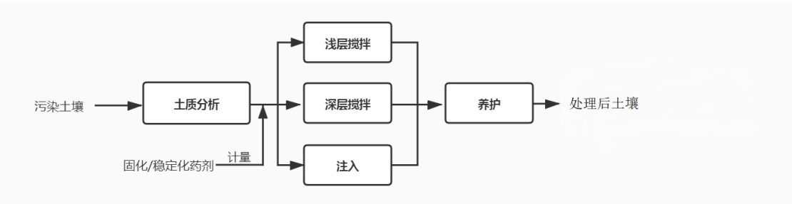
图1 原位固化/稳定化工艺流程图
